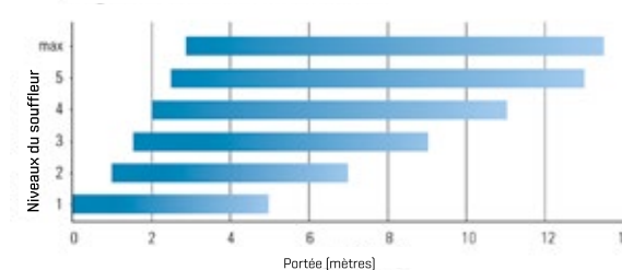
Portée en fonction de la vitesse du ventilateur
