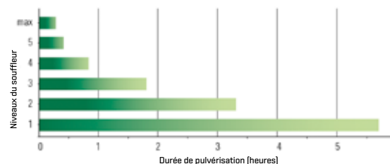
Temps de pulvérisation ASI200
